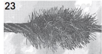
23 Brzdové lano jeřábu s dráždem. Všechny vnější dráty jsou vlivem opotřebování na výstupní hubici 1x na délku pletení polámané. Zlomené části se potom mačkaly do konečného bodu posunu.
