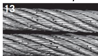
13 Zlámání drátů na ocelových lanech se zavřenými prameny způsobené vyčerpáním.
