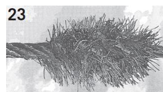
23 Brzdové lano jeřábu s držadlem. Všechny vnější dráty jsou vlivem opotřebování na výstupní hubici 1x na délku pletení poláhány. Zlomené části se potom mačkaly do konečného bodu posunu.
