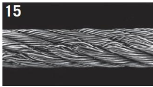
15 Toto lano bylo taženo přes okraj kladkostroje. Všimněte si stopy poškození.
