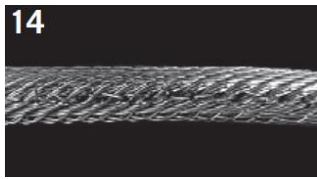
14 Toto nekroutivé ocelové lano bylo taženo přes okraj kladkostroje, a tím se hodně poškodilo.
